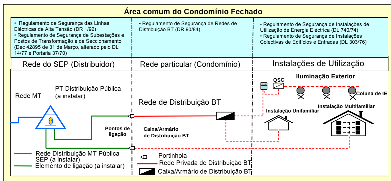
Figura 2 – Condomínio alimentado a partir de um PT (a edificar na área do empreendimento)
