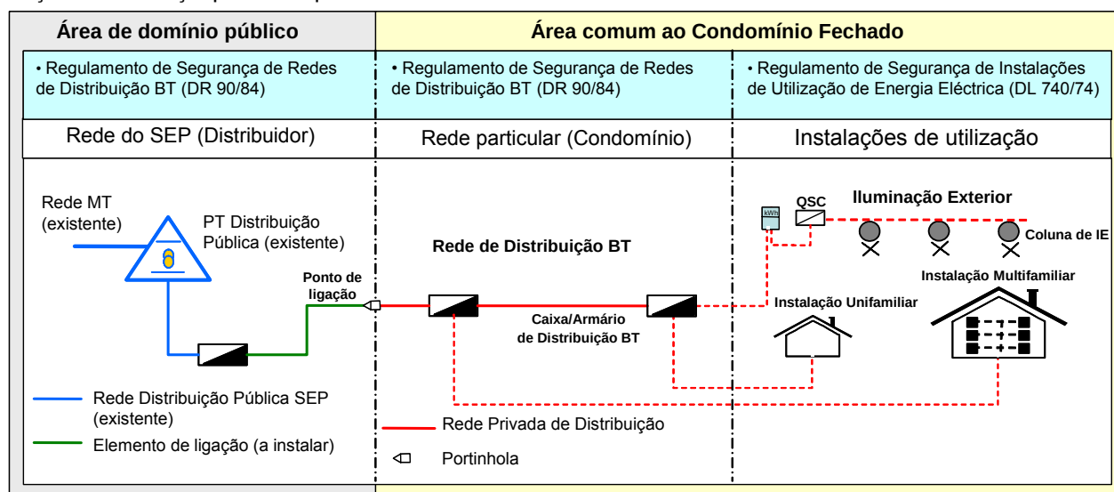
Figura 1 – Ponto de ligação: portinhola
